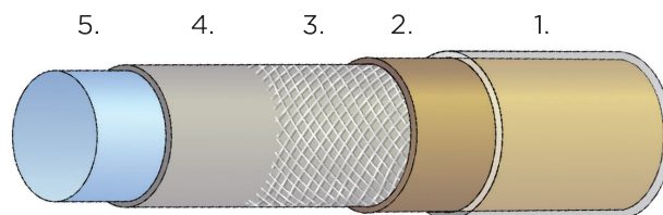
1.FluoroPEELZ® 2.Pebax® / ナイロン製被覆 3.LCP モノフィラメント 4.PTFE Sub-Lite-Wall® ライナー 5.PTFEマンドレル
